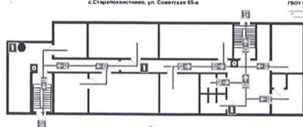
План эвакуации из помещений 1-го этажа ГБОУ СОШ с. Старопохвистнево, расположенный по адресу: Самарская обл., Повзневский р-он, с. Старопохвистнево, ул. Советская 65-а
